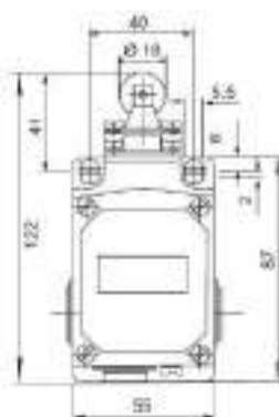
KLPRSO KLPRO
