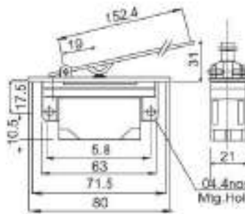
KLSILR1 KLSILR2
