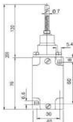
KLSCW
