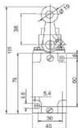
KLSL1
